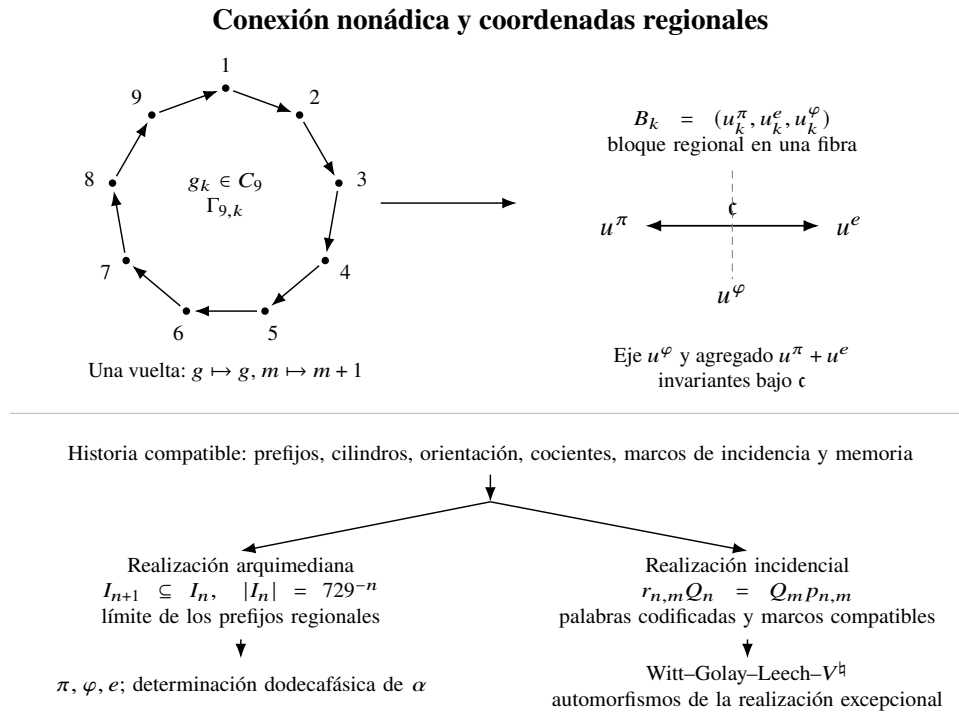
Figura 10.3: Nueve fases de una conexión y dos realizaciones de la historia compatible. El ciclo representa la fase; cada vuelta incrementa el contador. El diagrama regional representa la involución \mathfrak{c} , que intercambia clausura y propagación y fija el eje de autoescala en una fibra. Esta invariancia no impone que el eje sea constante durante el transporte. Las dos aplicaciones inferiores utilizan el mismo prefijo: una determina su límite numérico y la otra conserva palabras y marcos de incidencia. Los mapas de esta segunda realización se especifican en la sección 21.11.1; el recorrido excepcional se desarrolla después.
