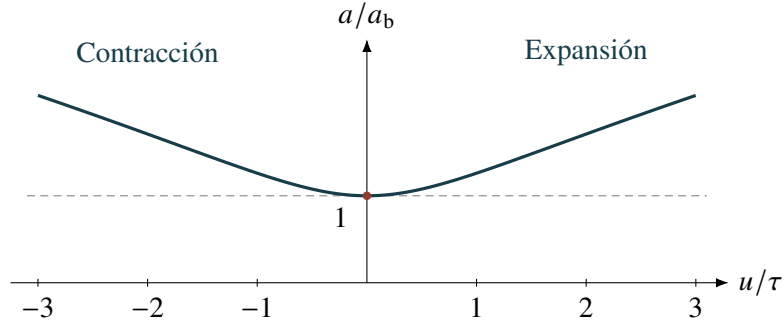
Figura 135.1: Perfil adimensional de la solución demostrada: a/a_b = (1 + (u/\tau)^2)^{1/3} . Los parámetros a_b y \tau se calculan desde \rho_0, s_0, G ; el dibujo representa toda la familia reescalada.
