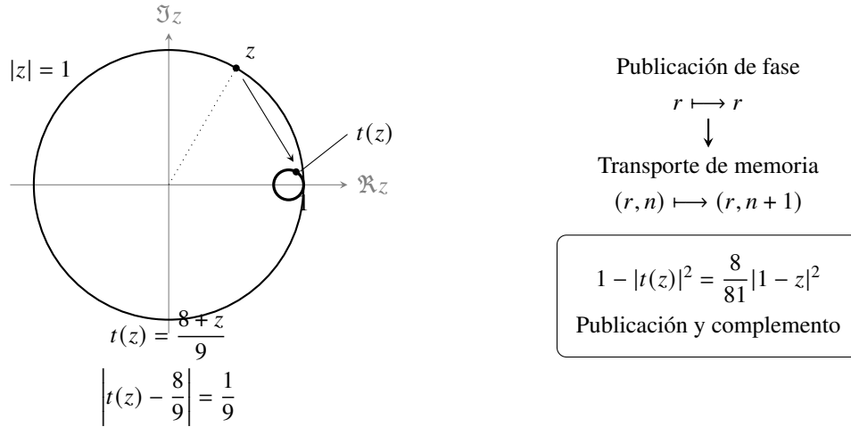
Figura 97.1: La carta circular de la compresión nonádica. A la izquierda, el círculo unidad y su imagen de centro 8/9 y radio 1/9 , dibujados a la misma escala; se muestra la imagen de z = e^{i\pi/3} . A la derecha, el retorno de fase se acompaña de avance de memoria. El balance inferior cuantifica la componente complementaria. Esta figura representa el mapa t , distinto del factor modal q = 5/9 de la carta central.
