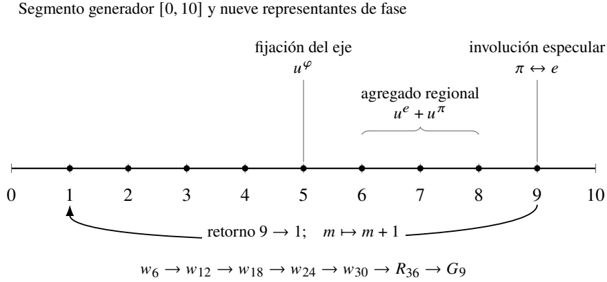
Figura 10.4: Representación rectilínea de la conexión noádica. La marca 5 sitúa la primera saturación fuerte y el eje regional de autoescala; la llave 6–8 identifica el agregado ternario fijado en cada fibra; la fase 9 selecciona la orientación de clausura. El retorno conserva la fase e e incrementa la memoria. Las abscisas numeran posiciones operativas, mientras las etiquetas u^\pi, u^e, u^\varphi designan bloques de \mathbb{F}_3^6 .
