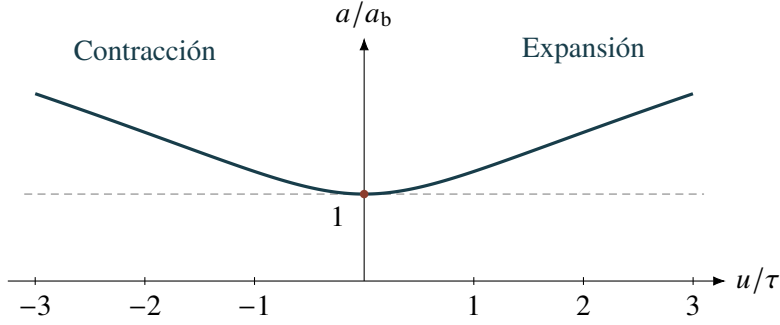
Figura 88.1: Perfil adimensional de la solución demostrada: a/a_b = (1 + (u/\tau)^2)^{1/3} . Los parámetros a_b y \tau se calculan desde \rho_0, s_0, G ; el dibujo representa toda la familia reescalada.
