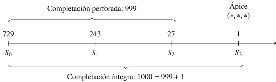
Figura 4.2: Estratos de la completación cúbica. La disposición representa la descomposición conjuntista, no una escala métrica. Los 243 elementos de S_1 son tres estratos coordenados de 81 elementos; los 27 de S_2 son tres estratos de 9. El ápice completa la partición.
