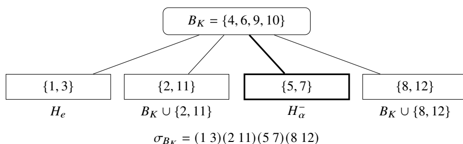
Figura 21.4: La estrella concreta de la bandera dodecafásica. Cada línea indica la unión de la cuaterna central con el par de su extremo; la línea gruesa señala la hexada seleccionada también por los signos anteriores al acarreo de \alpha . Los cuatro pares agotan las ocho posiciones exteriores.
