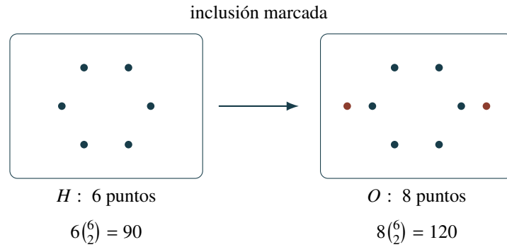
Figura 120.1: Incidencia marcada de seis a ocho puntos. El dibujo representa los conjuntos y la inclusión; no pretende convertir las caras o vértices de un cubo en bloques de Steiner sin su mapa de incidencia.
