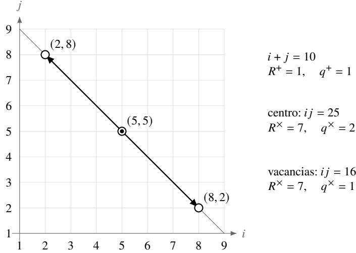
Figura 16.1: Centro electrónico y vacancias conjugadas en la carta APP. La diagonal es la fibra aditiva \mathcal{F}_{10} ; el centro es el punto fijo de (i, j) \mapsto (10 - i, 10 - j) . Los dos desplazamientos de módulo 3 conservan la suma y el residuo producto y reducen en una unidad el cociente multiplicativo. Las flechas representan las deformaciones sobre la fibra.
