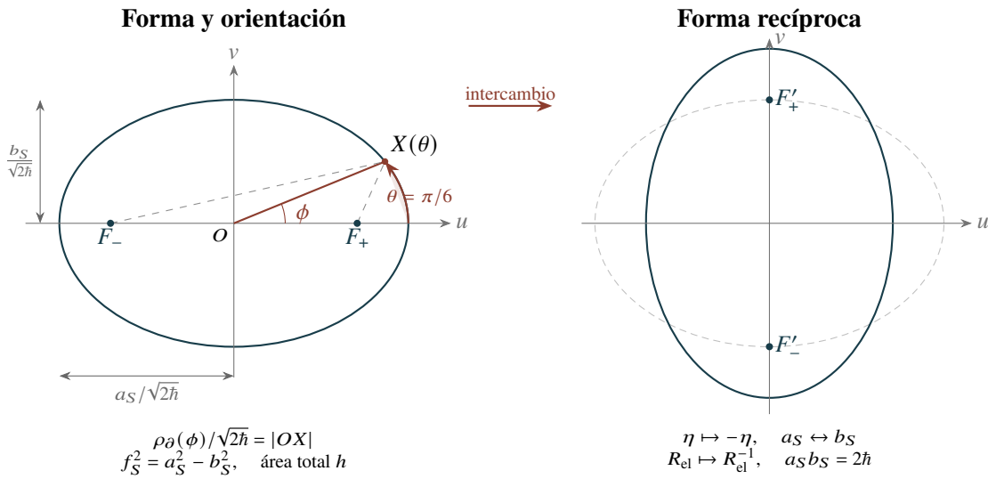
Figura 15.2: Semiejes, focos y reciprocidad de la elipse de acción en las coordenadas normalizadas u = Q/\sqrt{2\hbar} , v = P/\sqrt{2\hbar} . El sector marcado tiene fase paramétrica \theta = \pi/6 , distinta de su ángulo polar \phi ; su área de acción es \hbar\pi/6 . La figura utiliza el caso algebraico \xi = 1/3 para hacer legibles las relaciones: no atribuye ese valor a la salida angular HMT. Los focos se calculan desde los semiejes. A la derecha, el intercambio de ejes conserva el área total h e invierte el radio modular adimensional.
