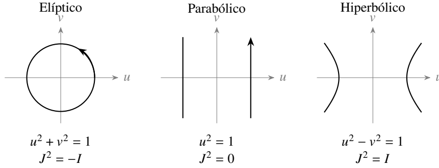
Figura 1.5: Realizaciones cuadráticas de TRIT. Para J_\tau = \begin{pmatrix} 0 & -\tau \\ 1 & 0 \end{pmatrix} , la exponencial conserva u^2 + \tau v^2 . La degeneración parabólica conserva u y transporta v linealmente. Los tres diagramas representan órbitas de formas cuadráticas; su tipo geométrico corresponde a la relación algebraica del generador.
