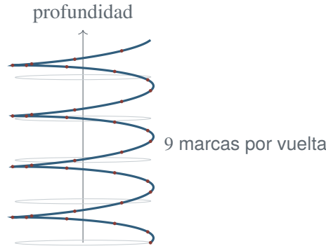
Figura 8.2: Hélice nonádica: los anillos son secciones de nivel; la curva conserva el avance de memoria.
