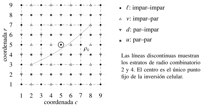
Figura 90.2: Clasificación sobre el atlas posicional. Las marcas distinguen las cuatro clases internas de paridad, anteriores a sus realizaciones físicas. La profundidad se mide con g(r, c) = \max(|r - 5|, |c - 5|) . La flecha ilustra (2, 3) \mapsto (8, 7) bajo la inversión celular; no representa una trayectoria dinámica ni un cambio de sabor. El círculo central marca (5, 5) , de profundidad cero.
