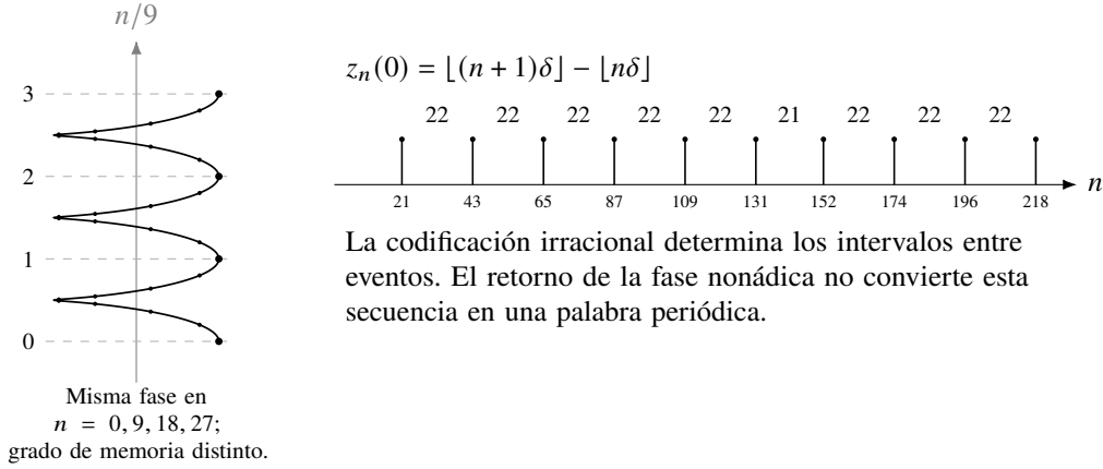
Figura 10.2: Representaciones complementarias del transporte. A la izquierda, proyección de la hélice (\cos(2\pi n/9), \sin(2\pi n/9), n/9) : el avance de nueve pasos recupera la fase e incrementa la altura. A la derecha, los diez primeros eventos de la palabra inferior para \delta = \log_{10}(10/9) , con separaciones exactas 21 o 22. La representación helicoidal no introduce una métrica física adicional.
