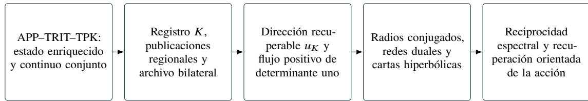
Figura 150.1: Dependencias de la ampliación. Las flechas representan composiciones especificadas en las demostraciones; la recuperación conserva las cartas y la orientación.
