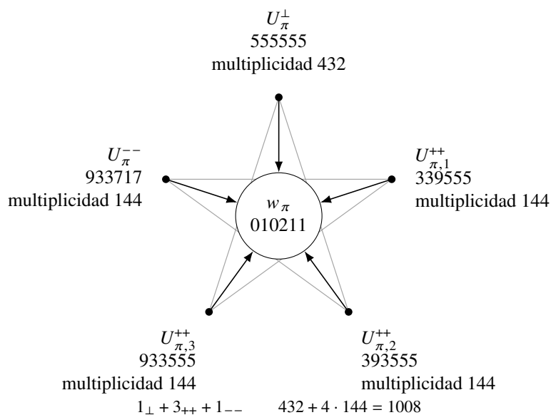
Figura 21.5: Las cinco regiones de \pi en disposición pentádica. Cada posición conserva su firma multiplicativa y su multiplicidad; las flechas radiales representan la proyección común \Psi(U) = 010211 . El contorno estrellado organiza las cinco posiciones de la carta. Su realización en las cinco octadas de Witt se efectúa mediante el alineamiento regional y la descomposición 4 + 1 del texto.
