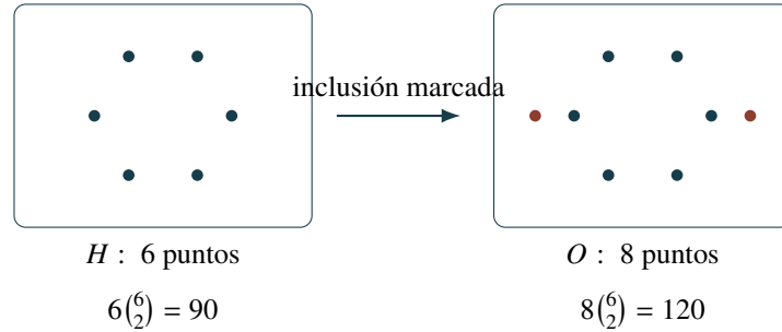
Figura 15.1: Incidencia marcada de seis a ocho puntos. El dibujo representa los conjuntos y la inclusión; no pretende convertir las caras o vértices de un cubo en bloques de Steiner sin su mapa de incidencia.
