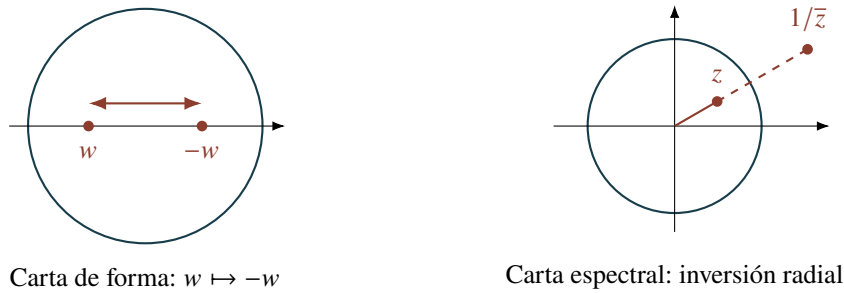
Figura 152.1: Dos reciprocidades tipadas. La primera permanece dentro del disco y transporta la orientación de la forma; la segunda intercambia el interior y el exterior del círculo unidad. Las posiciones dibujadas son esquemáticas.
