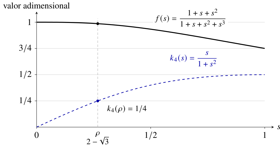
Figura 41.1: Respuesta constitutiva y núcleo del momento orientado. La curva continua es f y la discontinua es k_4 = \mathcal{D}^2 C_2 ; ambas se relacionan mediante (41.19). La recta vertical marca la sección de Pell, sin identificarla con los argumentos constitutivos s_+ o s_- .
